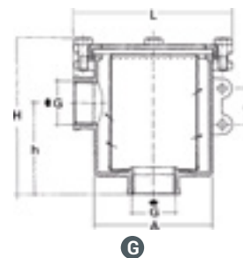
Support filtre Réf. 1460S (pour 1158 et 1160)
