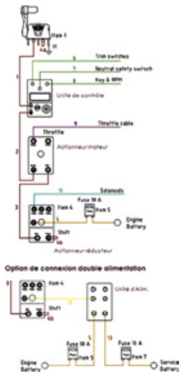
Installation électronique
