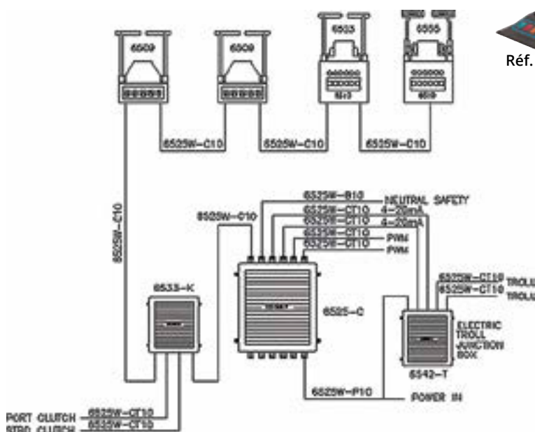
Exemple d'installation : 4 boîtiers commandes, 2 moteurs en PWM et 2 Trolling valve.
