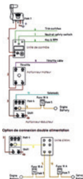
Installation électronique
