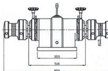
GH 1002 H Dimensions en mm
