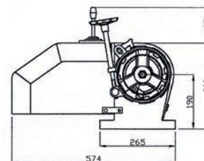
GH 1001 H Dimensions en mm
