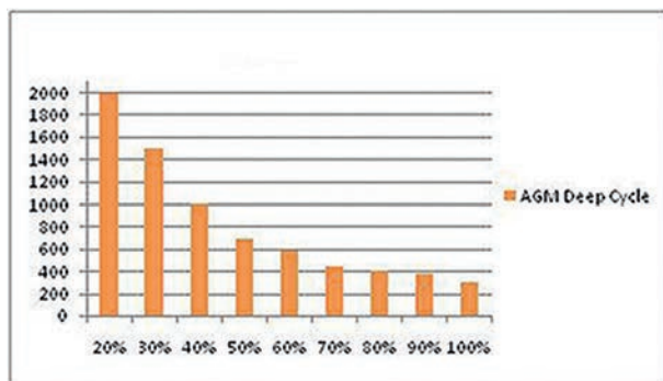
Durée de vie en cyclage Nombre de cycles / % de décharge
