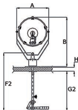
Commande en timonerie : montage C
