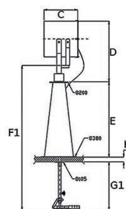
Commande en timonerie : montage C
